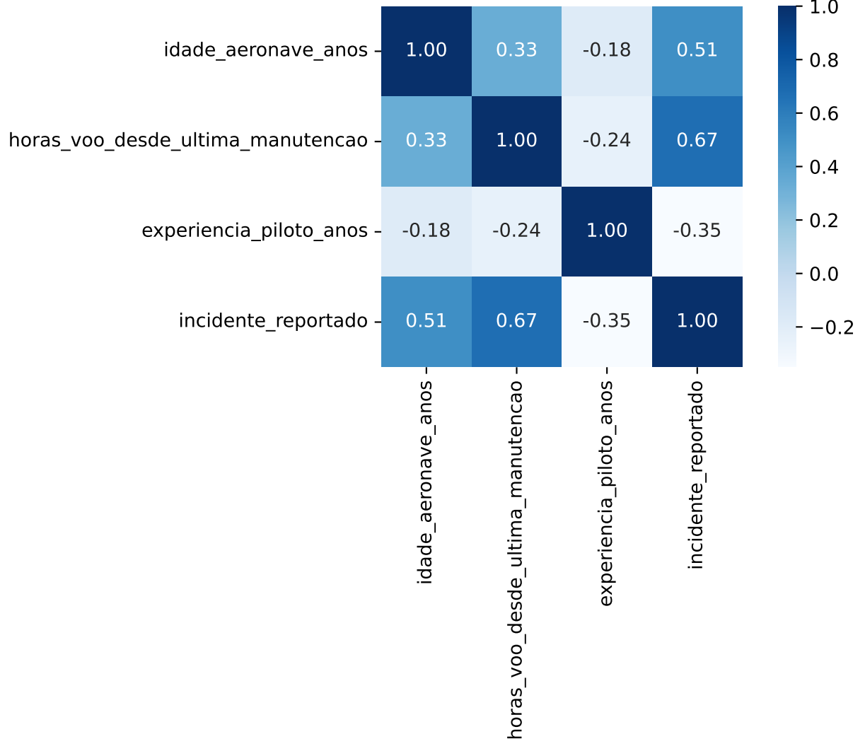
Correlações entre variáveis numéricas e alvo
